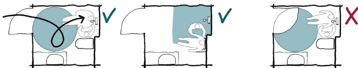
Figur: Eksempler med manøvreplads i bade- og wc-rum, plads ved siden af wc og i bruseområde.
